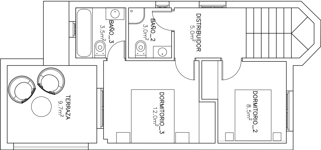
PLANTA PRIMERA
